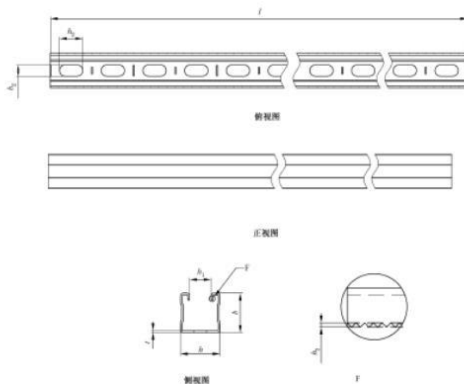
图 1 C形槽钢示意图
